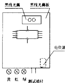
图2 黑线光藕板图
