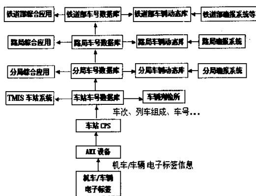
图1 ATIS 系统信息流程图
